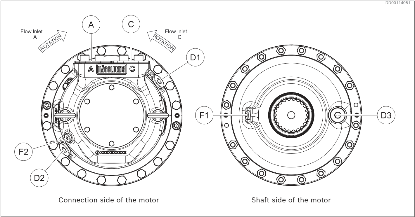
Fig. 3: Port connections Hägglands Atom
