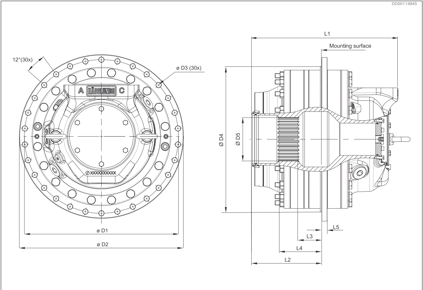
Fig. 59: Atom 30 C (center flange)
