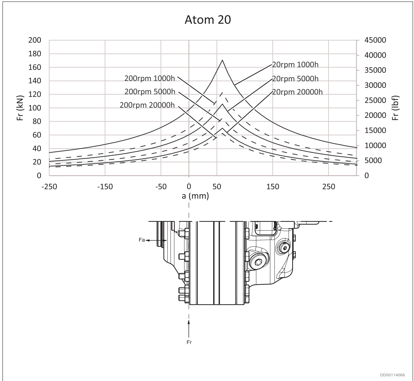
Fig. 32: Permissible external dynamic load Hägglands Atom 20
