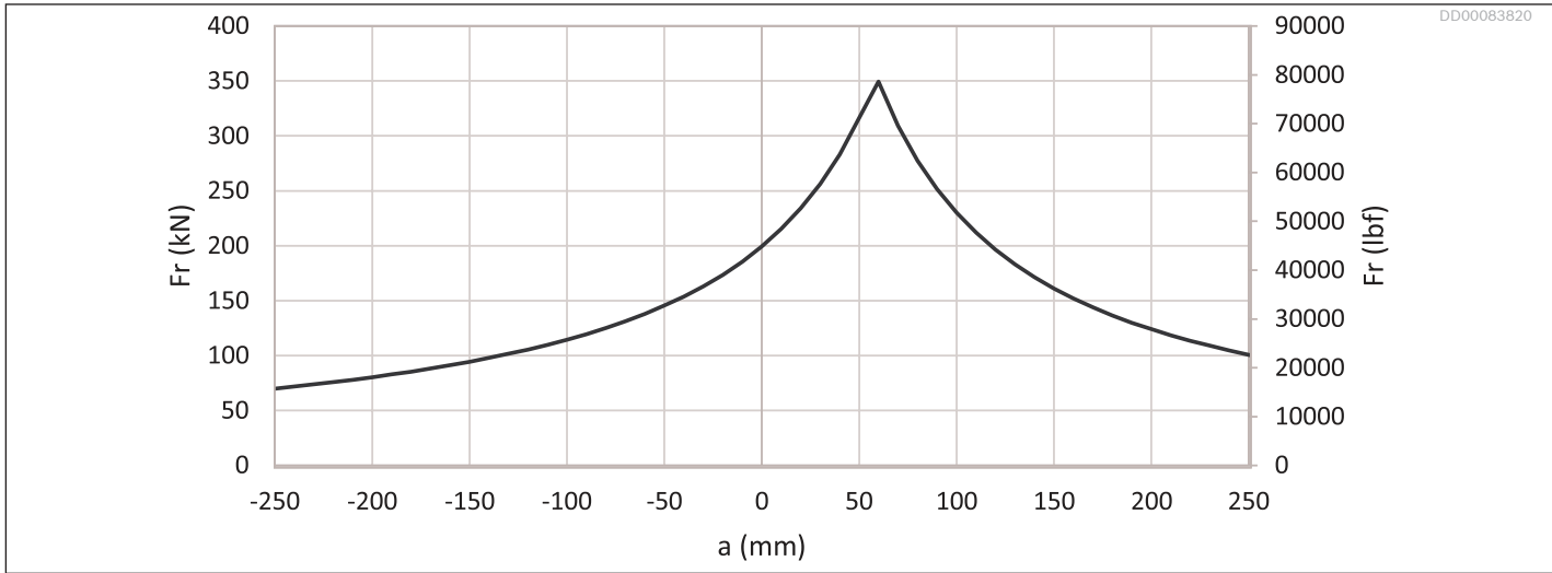
Fig. 37: Permissible external static load Hägglands Atom 20
