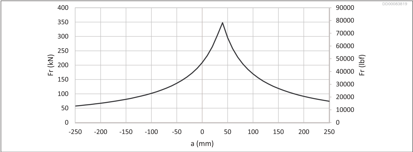
Fig. 36: Permissible external static load Hägglands Atom 10
