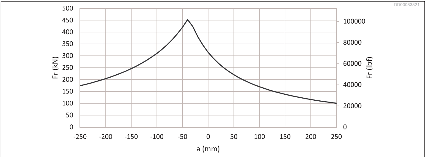
Fig. 38: Permissible external static load Hägglands Atom 30 C (center flange)
